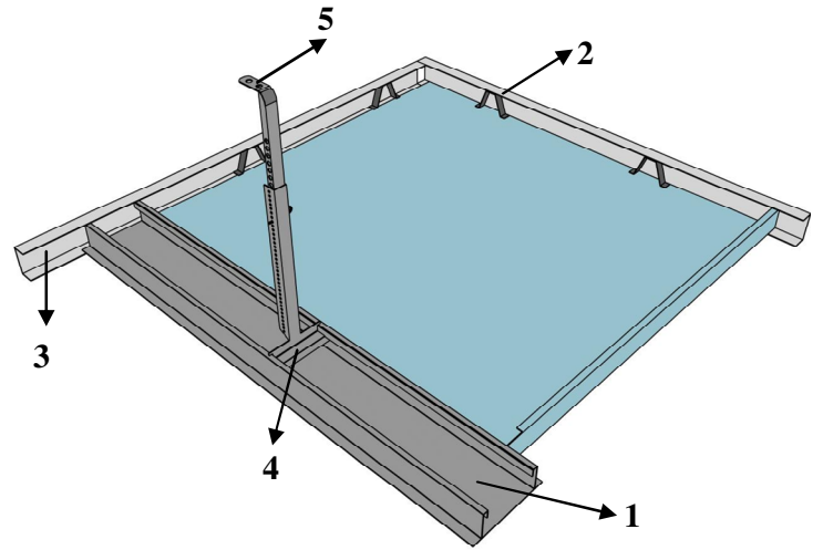
SİSTEM DETAYI
